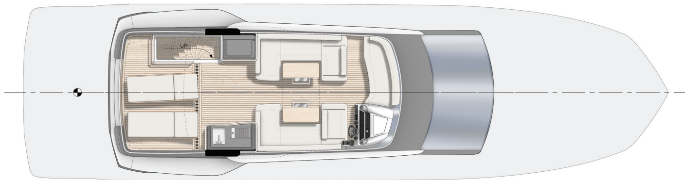
FLYBRIDGE
