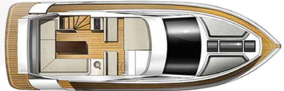
FLYBRIDGE
